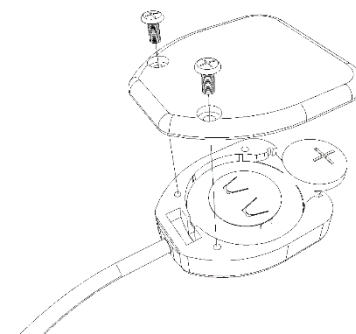
Abb. 2: VarioMobil PLUS schematische Darstellung
